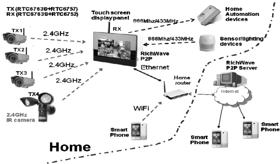
物聯網之智慧家庭無線安防監控、家庭自動化及家庭燈控之應用環境
