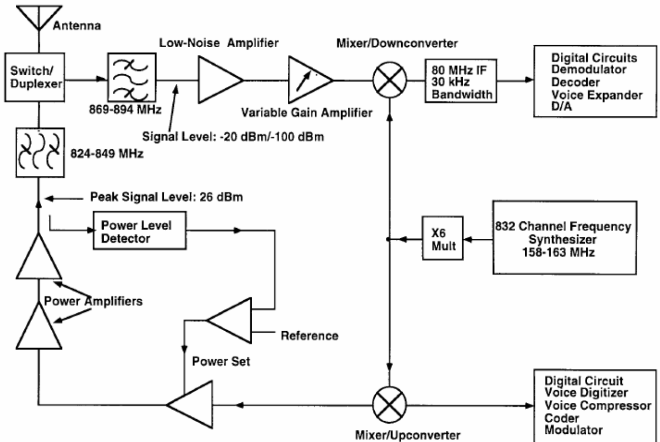
行動電話射頻簡易方塊圖
